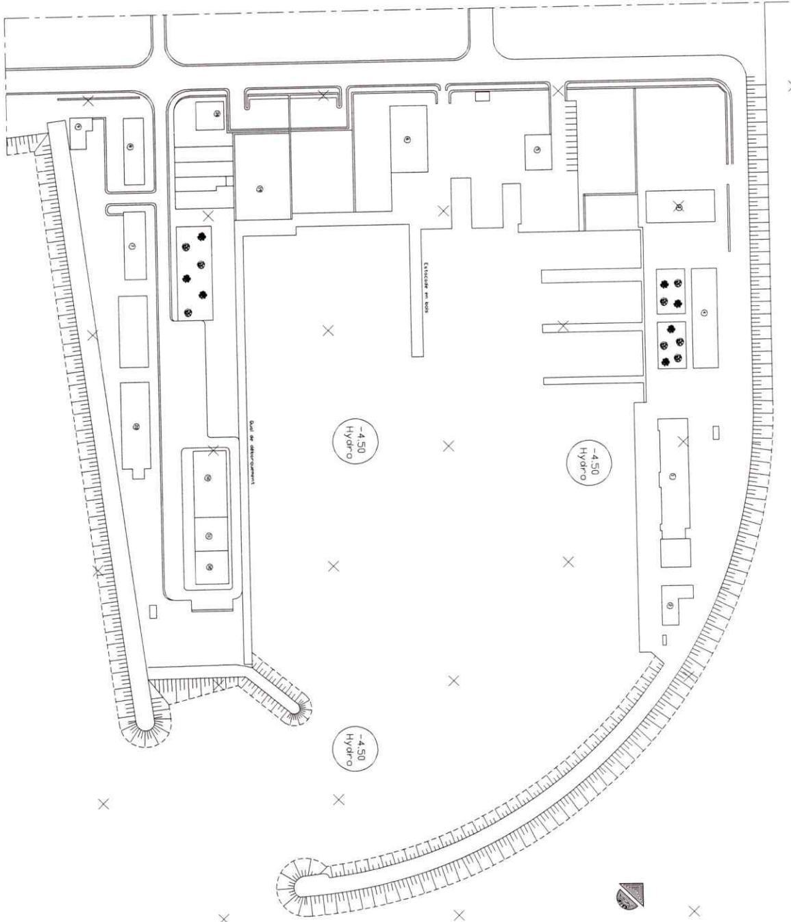
Plan masse du Port de Pêche de la GDULETTE
